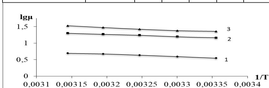
Рисунок 3. – График зависимости значения молярной электропроводности в водном растворе с акриловой кислотой и акриламидом при 298-318К
