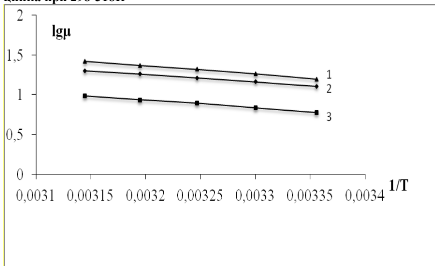
Рисунок 5. – График зависимости молярной электропроводности акриловой кислоты в водном растворе с добавлением железа, меди и цинка при 298-318К
