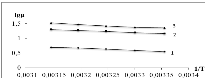
Расми 3. - Графики вобастагии чараёнгузарони молярӣ дар маҳлули обӣ бо кислотаи акрилат ва акриламид дар ҳарорати 298-318K
