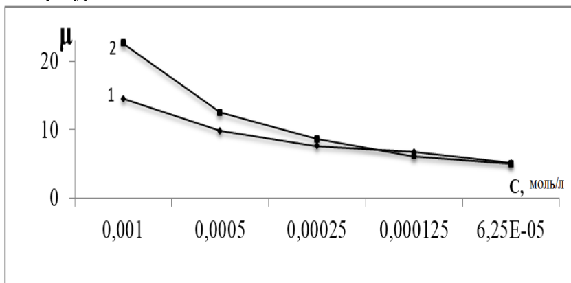
Рисунок 4. – График зависимости молярной электропроводности в воде от концентрации акриловой кислоты и акриламида при температуре 298К
