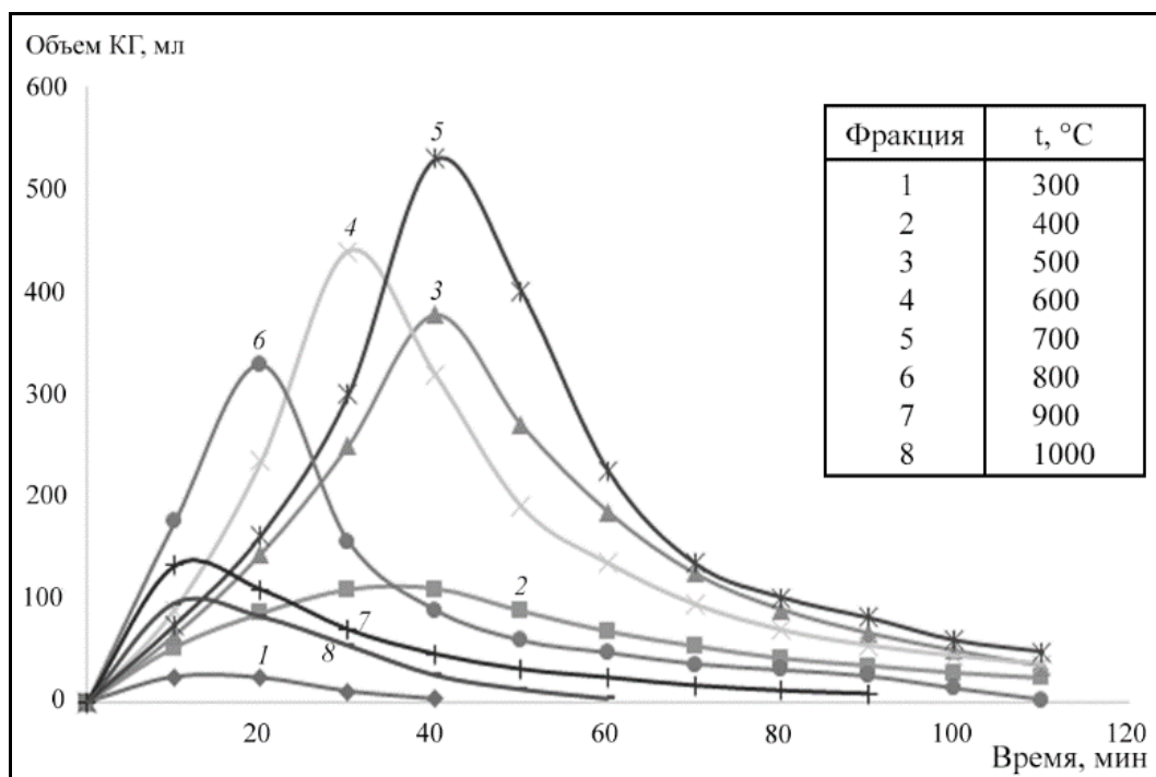
Рисунок 4 - Объем выделившегося коксового газа для каждой из восьми фракций в зависимости от продолжительности процесса термолитиза.
