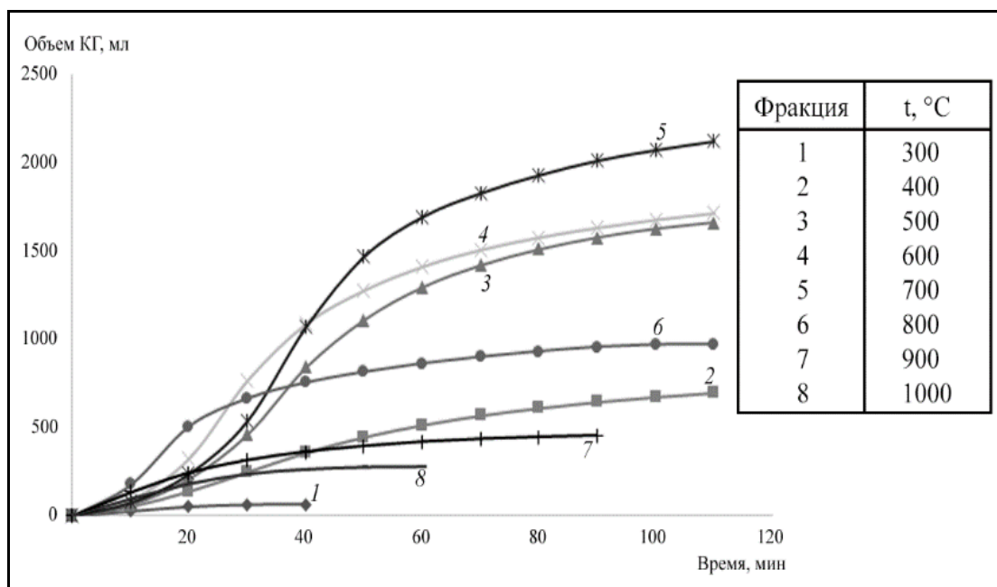
Рисунок 7 - Кинетические кривые накопления коксового газа в восьми фракциях.
