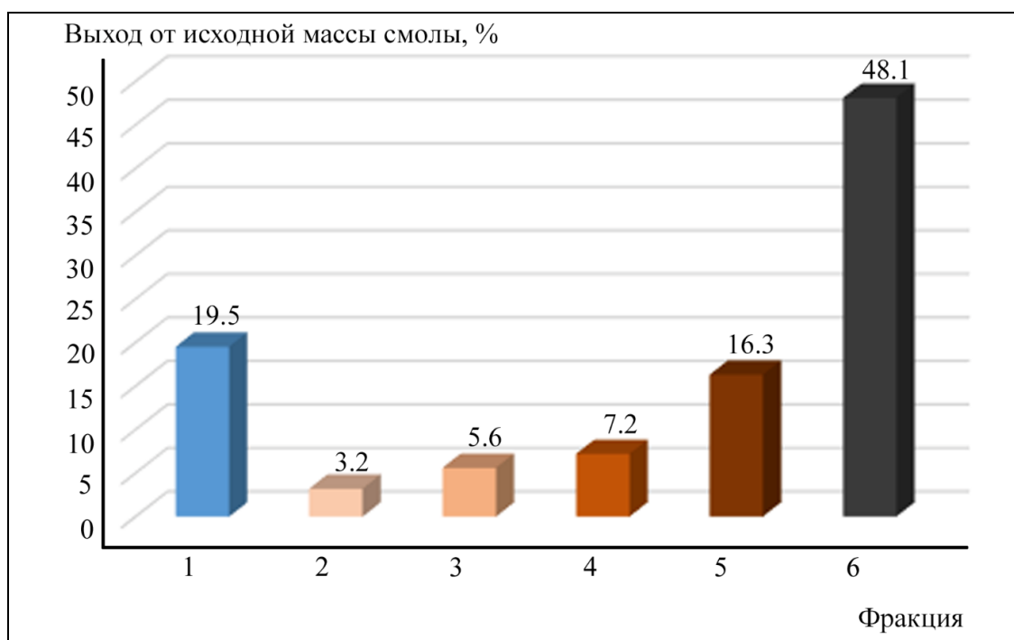
Рисунок 9 - Диаграмма по выходу легких фракций каменноугольной смолы (в процентах от исходной массы смолы)
