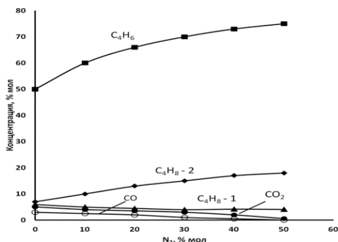
Рисунок 3.7. Влияние азота на выход компонентов в контактном газе процесса превращения этанола в дивинил: 400^\circ\text{C} , объемная скорость по жидкому потоку \text{LHSV} = 6\text{ч}^{-1} , время контакта \tau = 0,5\text{-}1\text{с} , загрузка катализатора 10\text{ см}^3 , 0,8\% \text{H}_2\text{O}_2 в этаноле при использовании 30%-ного водного раствора пероксида водорода
