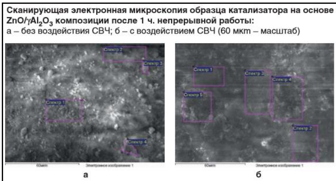
Рисунок 3.21. Сканирующая электронная микроскопия образца катализатора на основе \text{ZnO}/\text{Al}_2\text{O}_3 после 1 ч непрерывной работы
