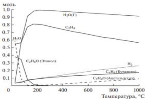
Рисунок 4.2. График температурной зависимости равновесного образования (моль) компонентов реакции
