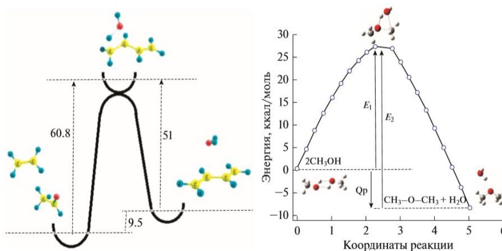
Рисунок 4.11. Поверхность потенциальной энергии реакции
