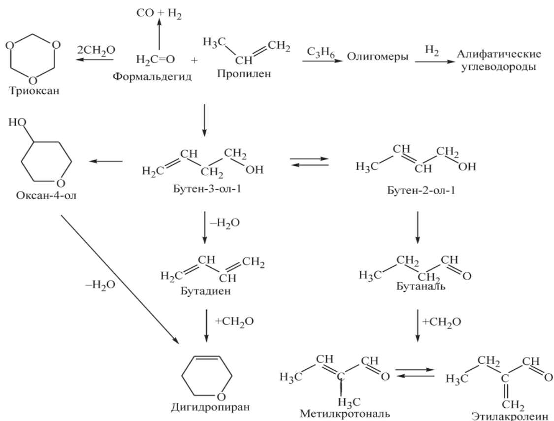
Схема 1.16. Маршруты образования C_4 углеводородов различных классов при Принс реакции
