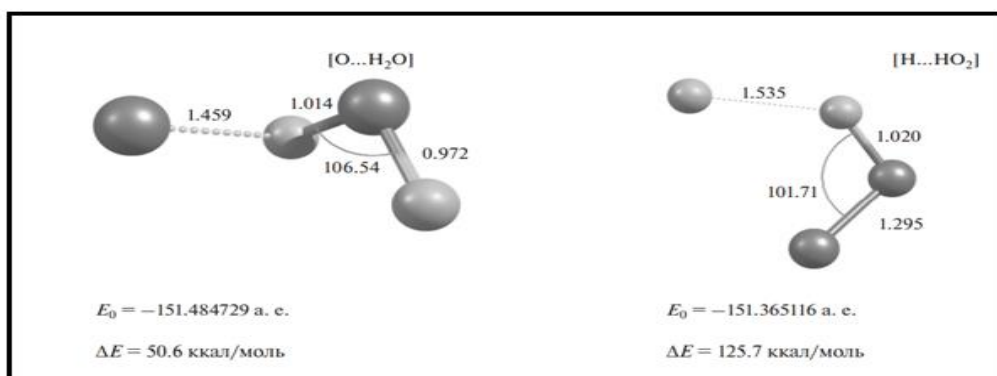
Рисунок 4.3. Энергии и геометрические параметры – межатомные расстояния (Å) и валентные углы – переходных состояний реакций разложения (3) и (4)
