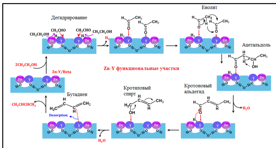
Схема 1.14. Механизм реакции превращения этанола в бутадие на бифункциональном Zn-Y/бета катализаторе
