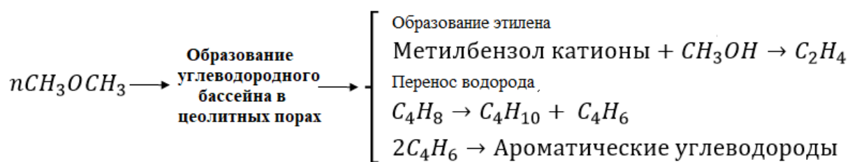
Схема 1.12. Образование аренов из ДМЭ
