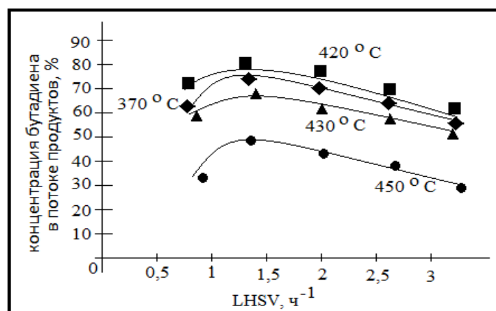
Рисунок 1.5. Зависимость концентрации от объемной скорости
