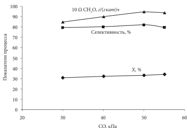
Рисунок 3.3. Влияние начальной концентрации метанола на процесс его дегидрирования в формальдегид при 850 °C, времени контакта 0.1 с, 1% H_2O_2
